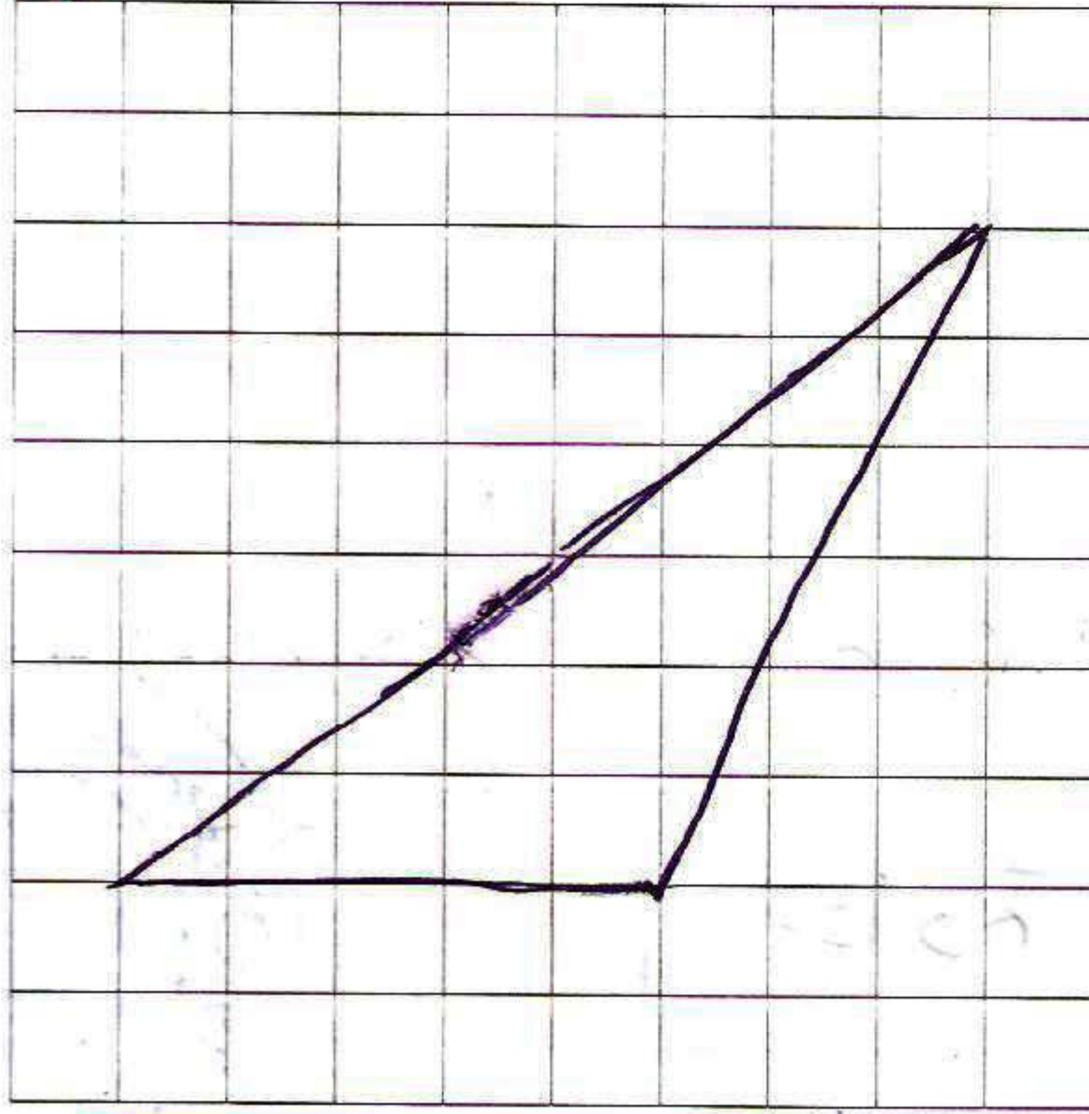
مثلث منفرج الزاوية
